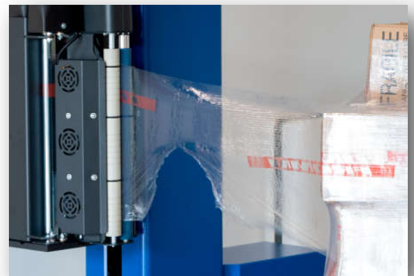
Taglio automatico del film, fine del ciclo di avvolgimento
